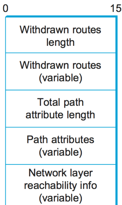
BGP-4 update packet format.
