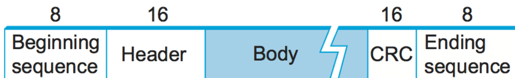
HDLC frame format.
