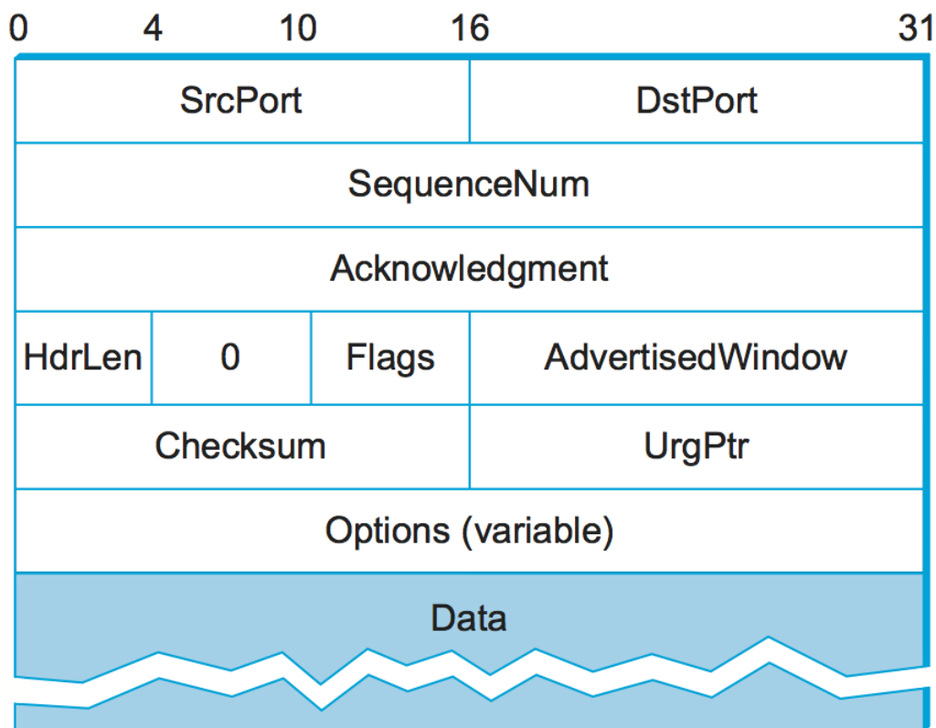
TCP header format.
