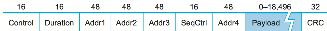
802.11 frame format.
