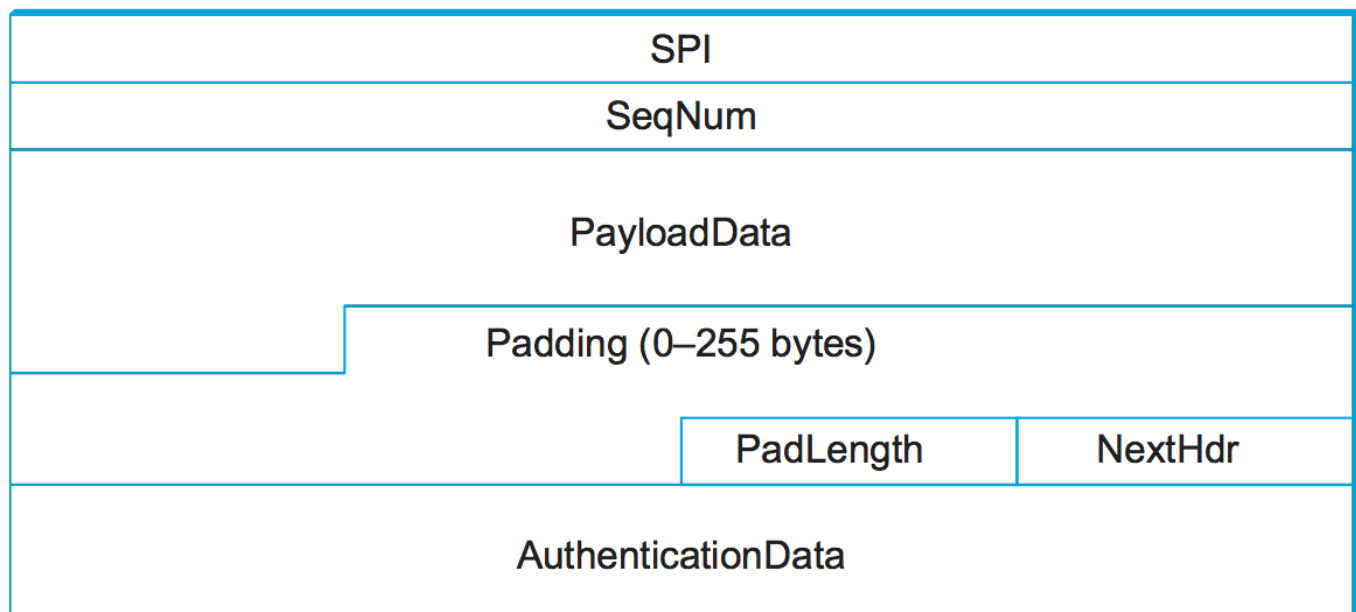
IPSec's ESP format.
