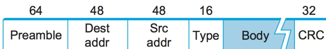
Ethernet frame format.
