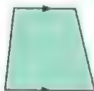
trapezium
