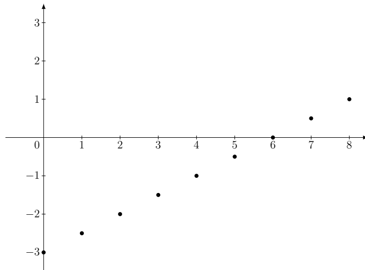
FIGURE 28.1 – Représentation graphique de la suite (u_n) tel que u_n = \frac{1}{2}n - 3
