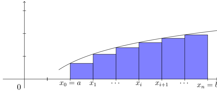
FIGURE 38.1 – Représentation graphique de AR_n
