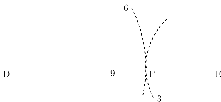
FIGURE 15.3 – Cas d'un triangle aplati
