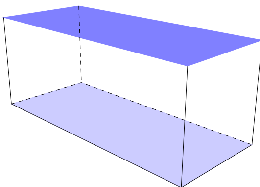
FIGURE 16.3 – Parallélépipède rectangle
