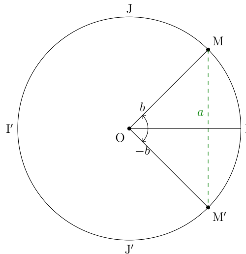
FIGURE 39.2 – Résolution de l'équation \cos(x) = a
