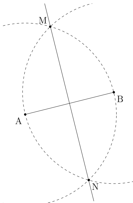
FIGURE 21.1 – Construction d’une médiatrice à la règle et au compas
