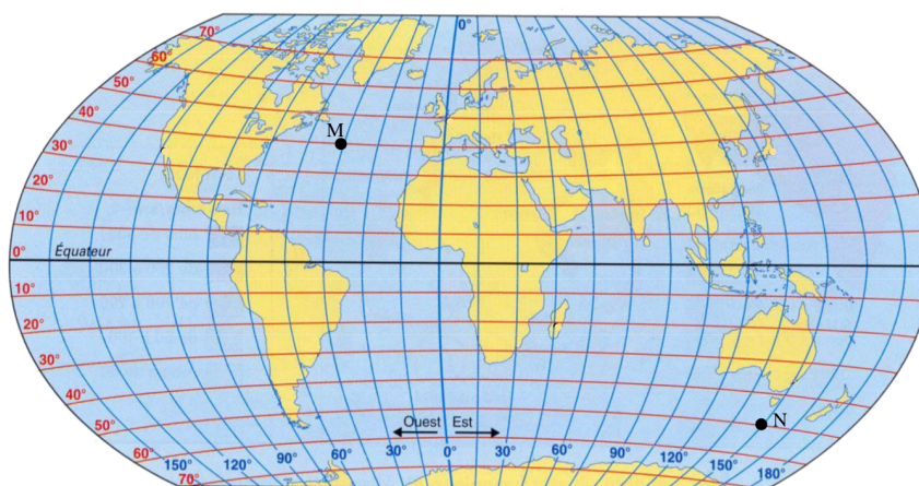
FIGURE 12.11 – Planisphère de l'exemple 12.11
