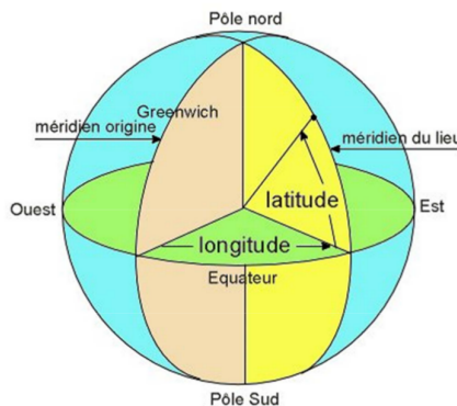
FIGURE 12.5 – Vocabulaire sur le planisphère (repérage sur une sphère)
