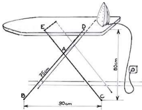
FIGURE 22.7 – Table à repaser, version CAPES
