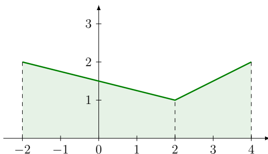
FIGURE 17.25 – Représentation graphique de la fonction f de l'exemple 17.53
