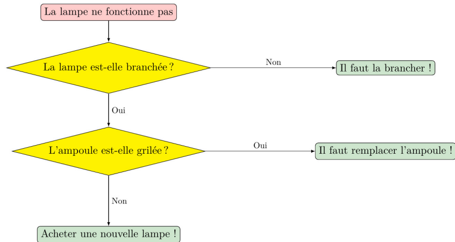
FIGURE 41.1 – Exemple d’algorithmes
