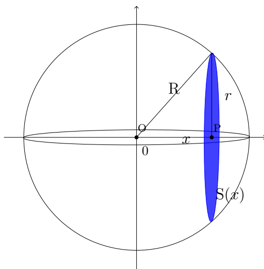
FIGURE 17.20 – Figure de la démonstration TS
