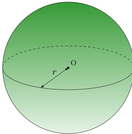
FIGURE 16.15 – Sphère de centre O et de rayon r
