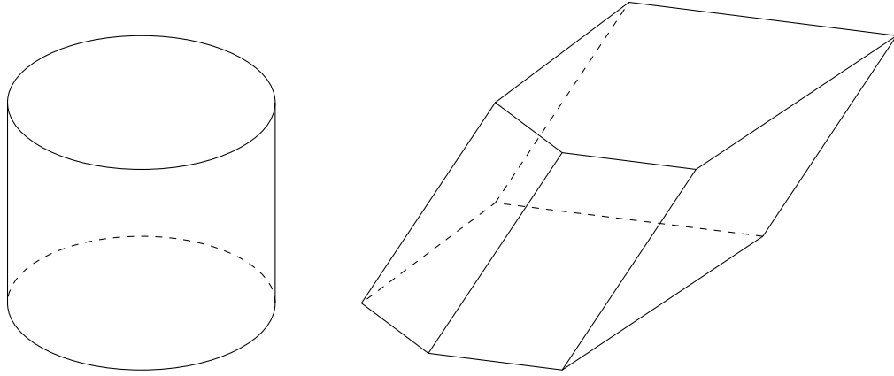
FIGURE 16.7 – Cylindre (à gauche) et prisme droit (à droite)
