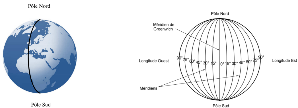
FIGURE 12.7 – Représentation de la planète Terre (à gauche) et de ses méridiens (à droite)
