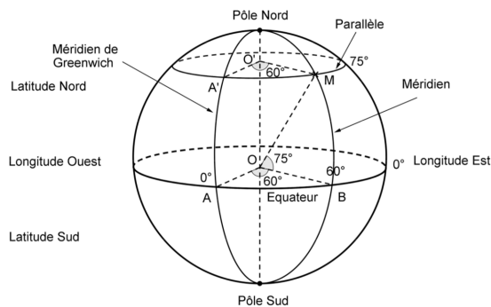
FIGURE 12.10 – Le point M se situe à l'intersection du 75° parallèle-nord ( \widehat{BOM} = 75^\circ ) et du 60° méridien-est ( \widehat{AOB} = 60^\circ ).
