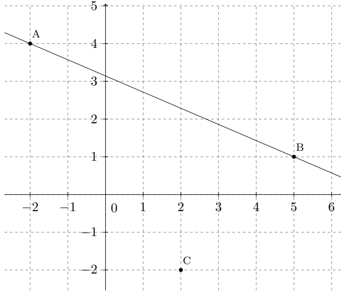
FIGURE 12.4 – Calcul de la distance du point C par rapport à la droite (AB)
