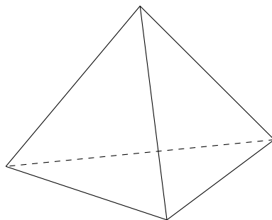
FIGURE 16.13 – Tétraèdre
