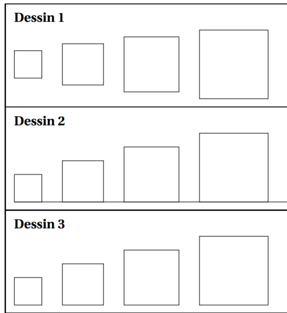
FIGURE 41.6 – Résultats possibles
