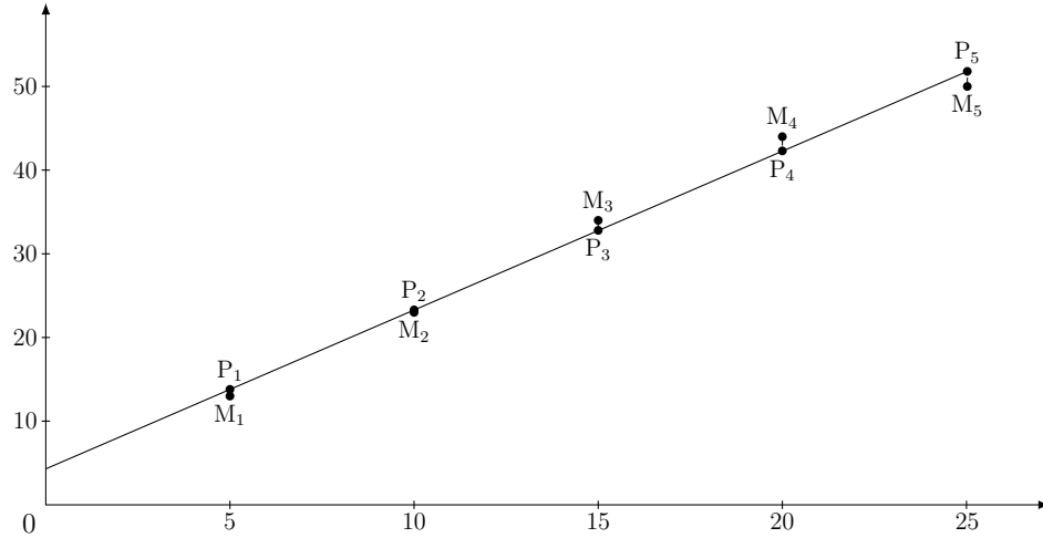
FIGURE 5.7 – Droite d'ajustement affine du nuage de points obtenue à l'aide de la méthode des moindres carrés
