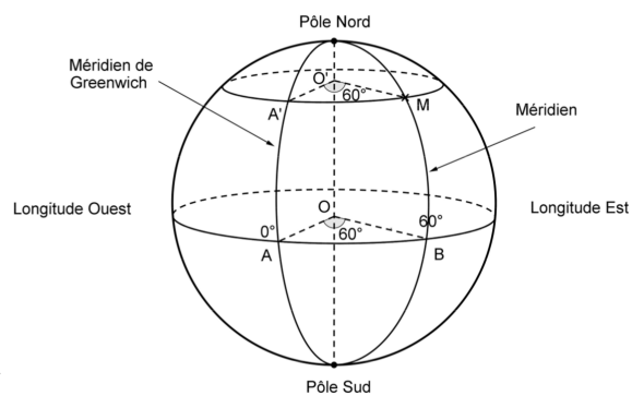
FIGURE 12.6 – La longitude du point M est représentée par la mesure des angles \widehat{AOB} et \widehat{A'O'M} où le point O est le centre de la Terre
