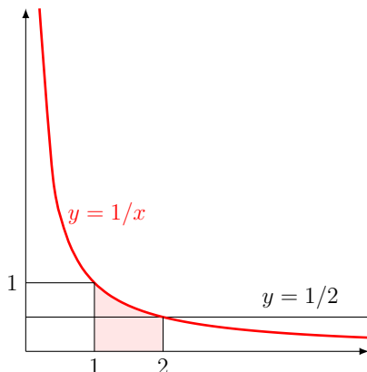
FIGURE 37.13 – Intégrale et inégalité
