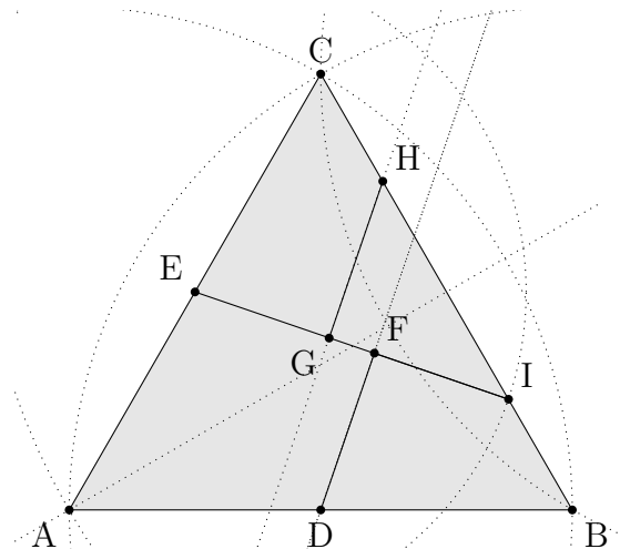
FIGURE 17.4 – Découpage de Dudeney (1902)
