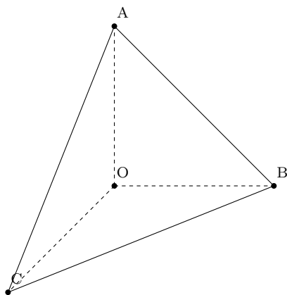
FIGURE 13.6 – Résultat de Descartes
