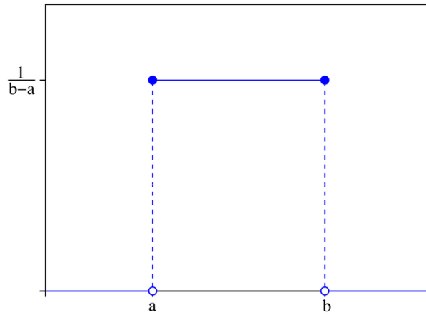
FIGURE 4.1 – Densité de la loi uniforme \mathcal{U}([a; b])
