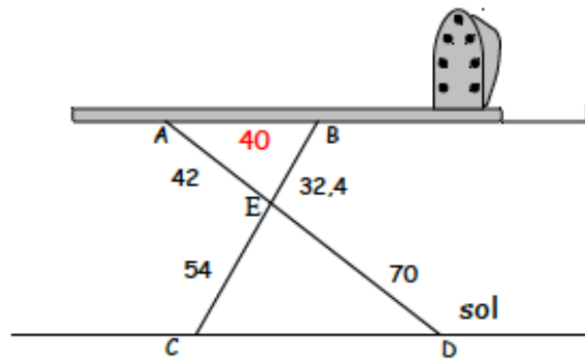
FIGURE 22.6 – Table à repasser, version brevet
