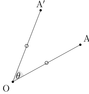
FIGURE 14.5 – A' est l'image par la rotation de centre O , d'angle \theta et dans le sens direct
