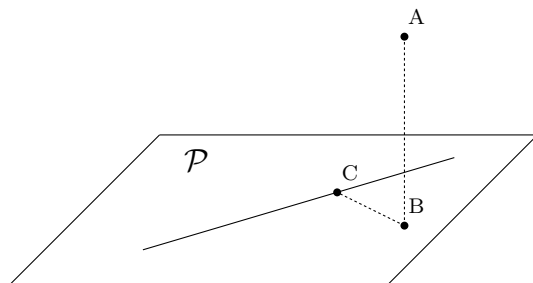
FIGURE 13.5 – Théorème des trois perpendiculaires
