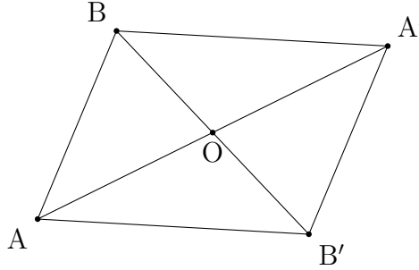
FIGURE 14.4 – Si s_O(A) = A' et s_O(B) = B' alors \overrightarrow{A'B'} = \overrightarrow{BA} = -\overrightarrow{AB} , c'est-à-dire que ABA'B' est un parallélogramme de centre O . Ainsi, A'B' = AB et (A'B') \parallel (AB) ; ce qui signifie que la symétrie centrale conserve les distances.
