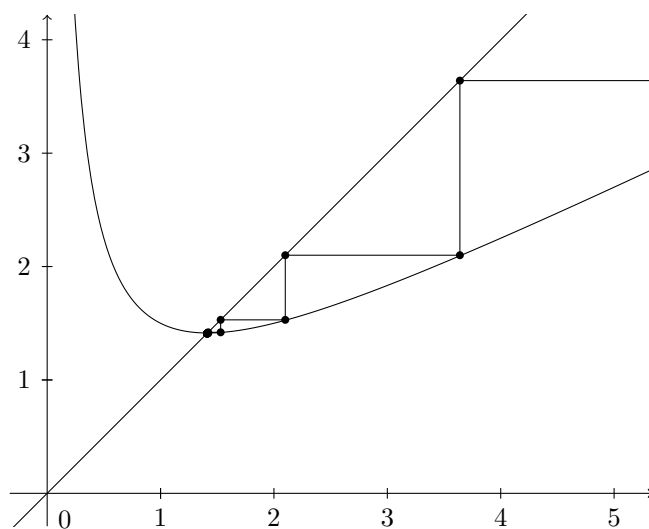
FIGURE 28.7 – Représentation graphique de la suite de Héron pour l'approximation de \sqrt{2}
