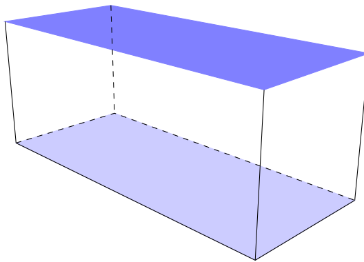
FIGURE 17.14 – Parallélépipède rectangle
