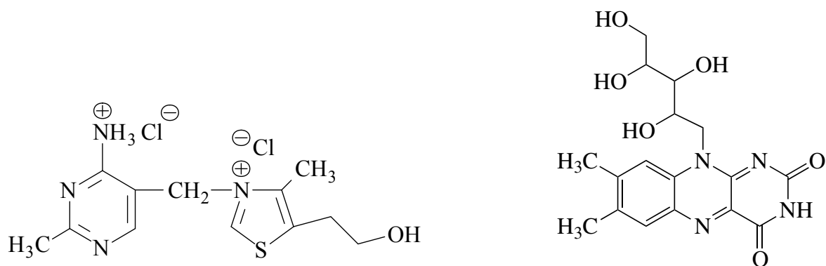
Thiamine – vitamine B1
