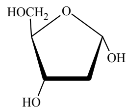
\alpha -2-D-désoxyribose (furanose)
