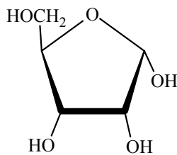
\alpha -D-ribose (furanose)
