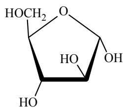
\alpha -D-arabinose (furanose)
