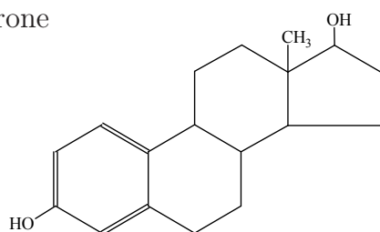
Estradiol ou œstradiol
