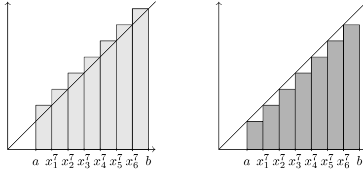
FIGURE 5.2: Les sommes de Darboux supérieures et inférieure de l'Exemple 5.7 (avec n = 7 ).
