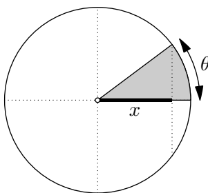
FIGURE 6.1: L'aire du secteur grisé est égale à \theta/2 .
