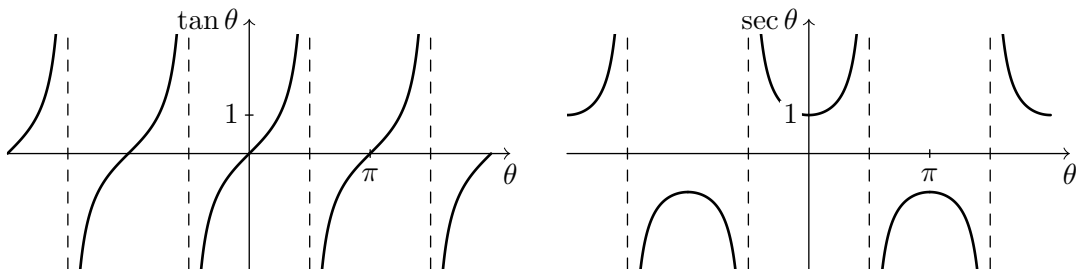
FIGURE 6.4: Les fonctions tan et sec.
