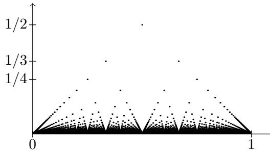
FIGURE 3.5: La fonction de Thomae, introduite dans l'Exercice 3.4, est discontinue en chaque rationnel, mais continue en chaque irrationnel.
