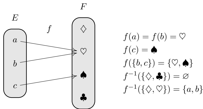
FIGURE 0.2: Une fonction f: \{a, b, c\} \rightarrow \{\diamond, \heartsuit, \spadesuit, \clubsuit\} .
