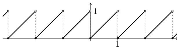
FIGURE 1.9: La fonction x \mapsto x - [x] est périodique, de période 1.
