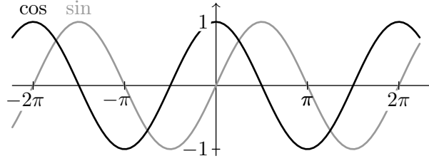
FIGURE 6.3: Les fonctions cos et sin.
