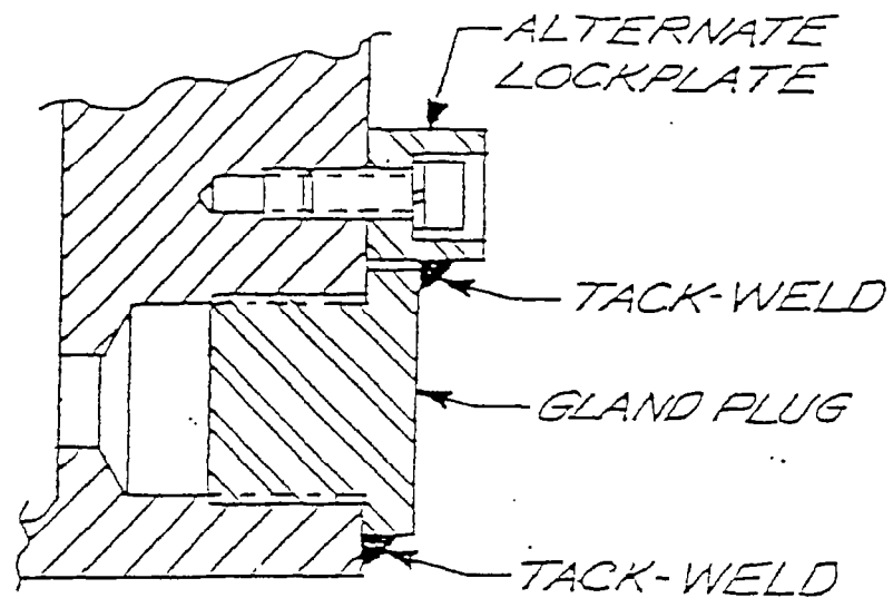
F I G U R E 4
